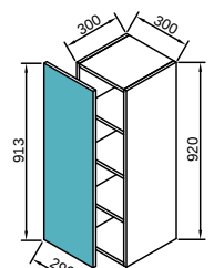
48 BΔ30 (навісна шафа 30)
