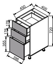
нижня тумба 40 три ящики
