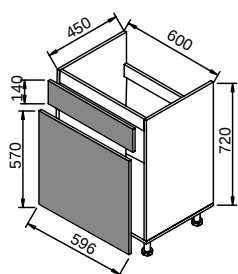
Нижня тумба мийка 60
