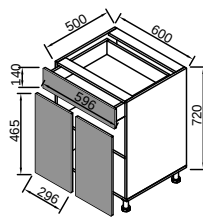
9 H60Ш1 (нижня тумба 60 з ящиком)
