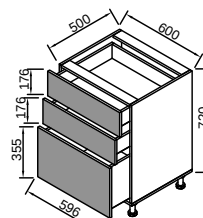
14 H60Ш3 (нижня тумба 60 на 3 ящика)
