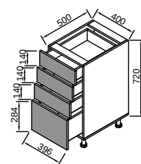
16 H40Ш4 (нижня тумба 40 на 4 ящики)
