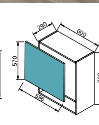
Навісна шафа сушка 60
