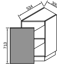
24 H330Y (нижня тумба 30 кутова)
