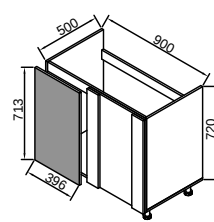
21 НМ95Ш (нижня тумба 90 під мийку щитова)
