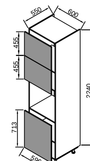
86 ШДД60 (шафа 60 під духовку)
