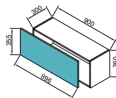
71 BM90 (навісна шафа 90 (360))
