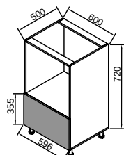
85 НД60Ш1 (нижня тумба 60 під духовку)
