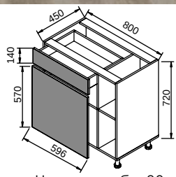
Нижня тумба 80 з ящиком і полицею. Універсальна
