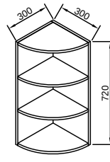
72 B30Y (навісна шафа 30 кутова відкрита)
