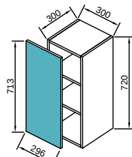
44 B30 (навісна шафа 30)
