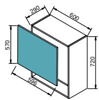
Навісна шафа сушка 60
