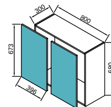
навісна шафа під сушку 80
