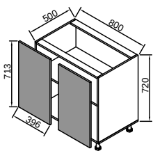
6 H80 (нижня тумба 80)
