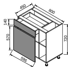
Нижня тумба 80 з ящиком і полицею. Універсальна
