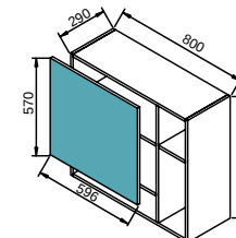
Навісна шафа 80 з полицею. Універсальна
