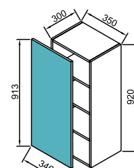
81 B35 (навісна шафа 35)
