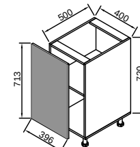
2 H40 (нижня тумба 40)
