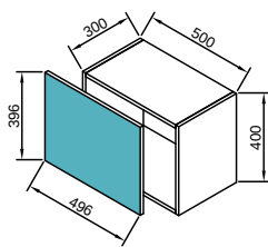
60 B50BT (навісна шафа 50 під витяжку)
