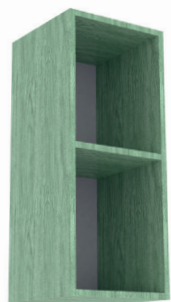
B-701 Шафа верхня без фасада 1 вставна поличка Висота - 720 мм Ширина - 200 / 300 / 400 / 500 / 600 мм Глибина - 300 мм
