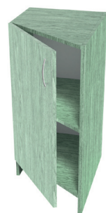
Н-805 Шафа нижня діагональна (закінчення) 1 фіксована полицка Висота - 820 мм Ширина - 300 мм Глибина - 570 мм
